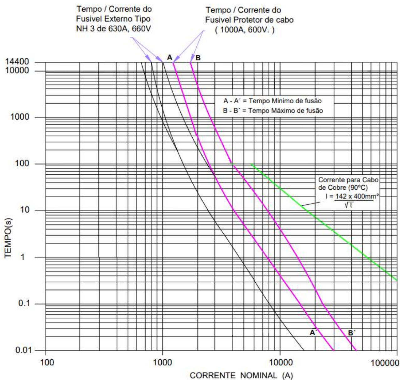
Figura 9 - Tempo Corrente de Fusível 630 A/gG (Bitola de cabo 400 mm² de cobre)
