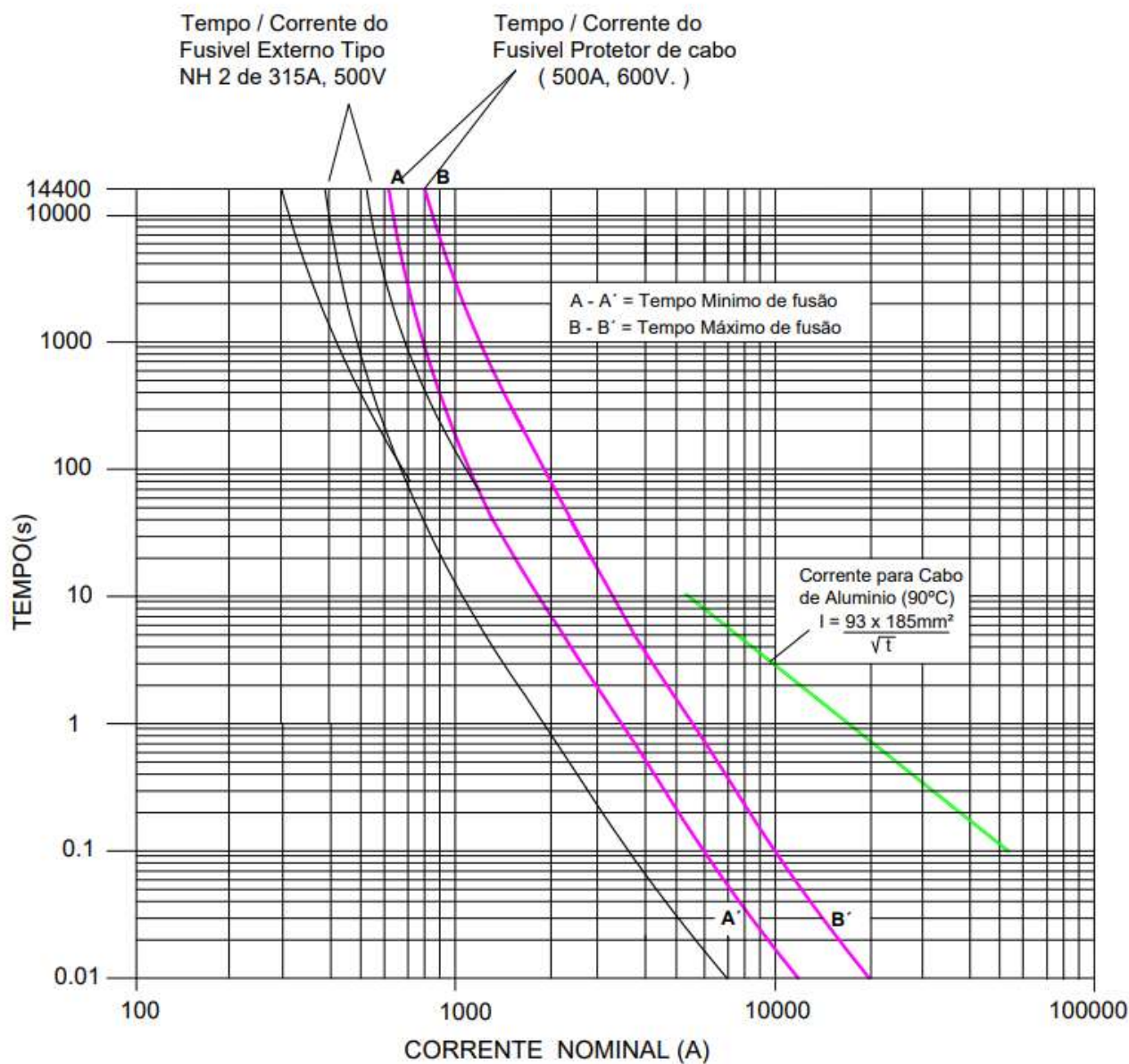
Figura 5 - Tempo Corrente de Fusível 500 A/gG (Bitola de cabo 185 mm² de alumínio)
