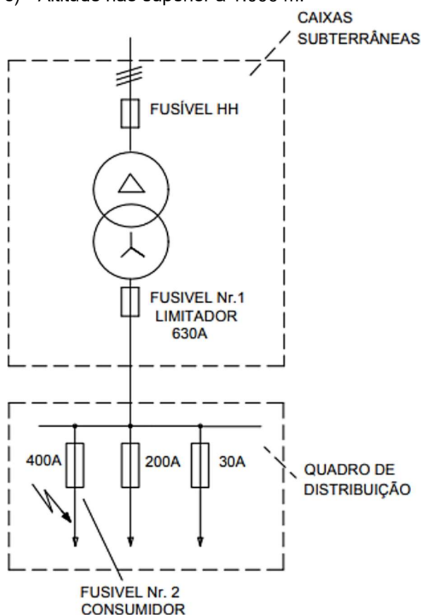
Figura 2 – Seletividade
